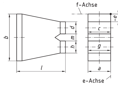
Hosenstück HS
